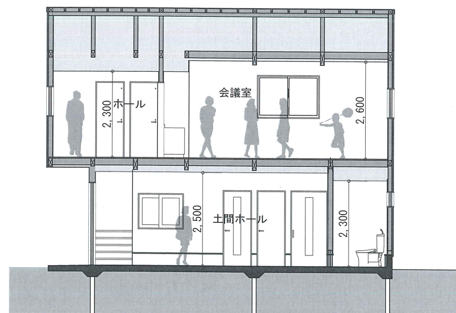
Y-Y断面図 1:100
