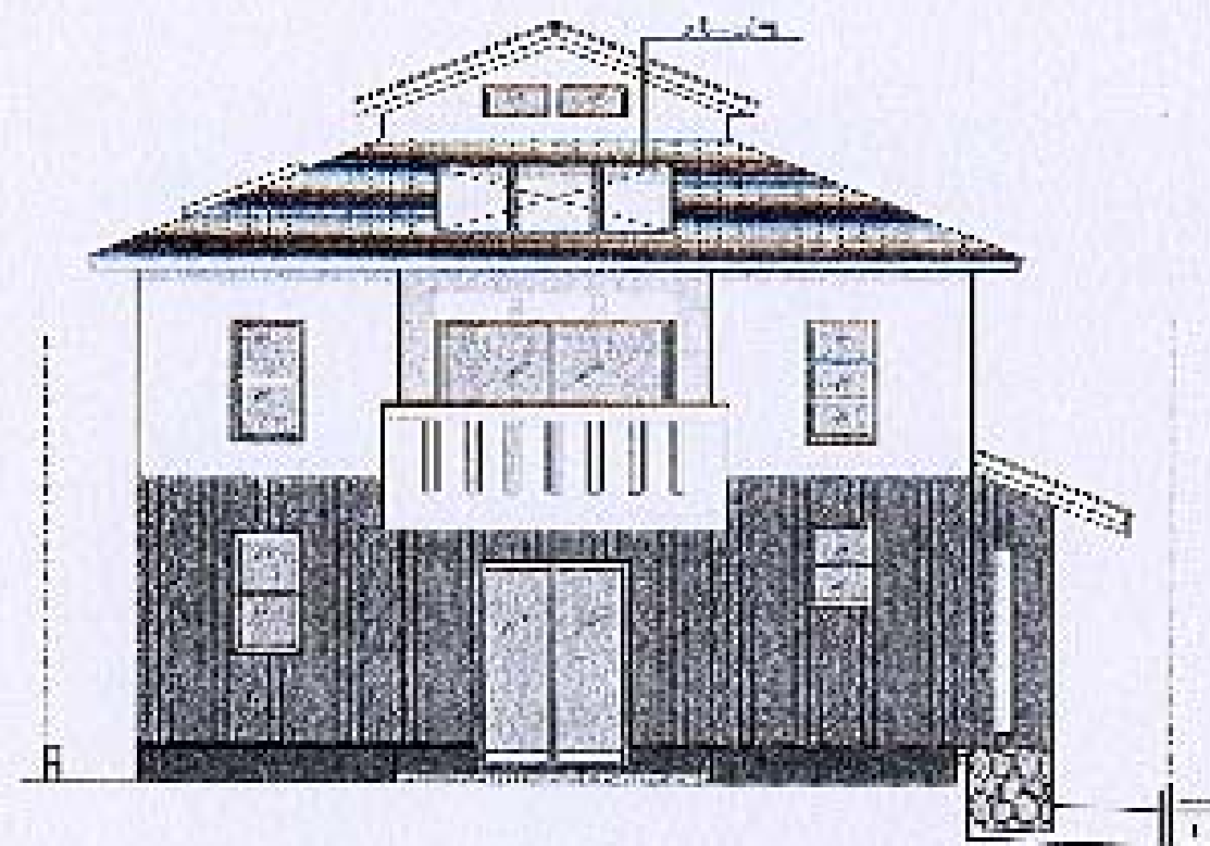
西側立面図
