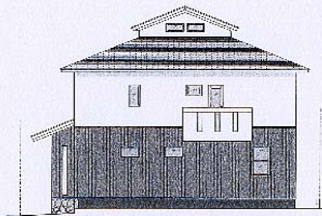
北側立面図
