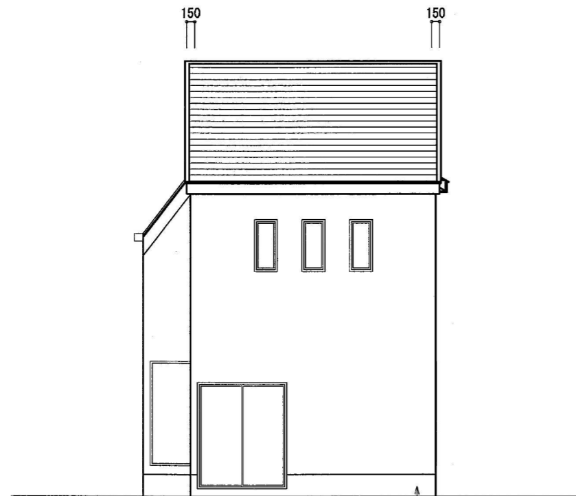
道路側 立面図 S:1/100
